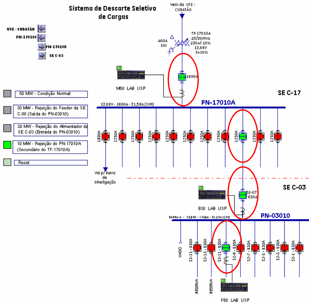
Figura 9 - Condição do ensaio de load shedding , no terceiro nível de prioridade.
